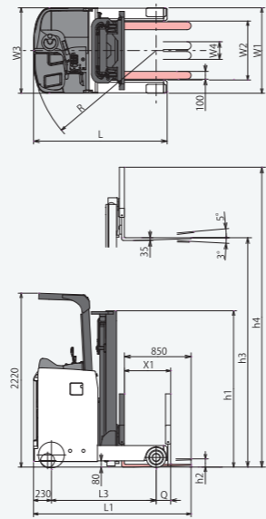
バッテリー前引出し仕様 1.4t~1.8t 積
