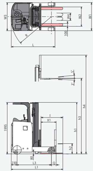
バッテリー前引出し仕様 0.9t~1.8t 積
