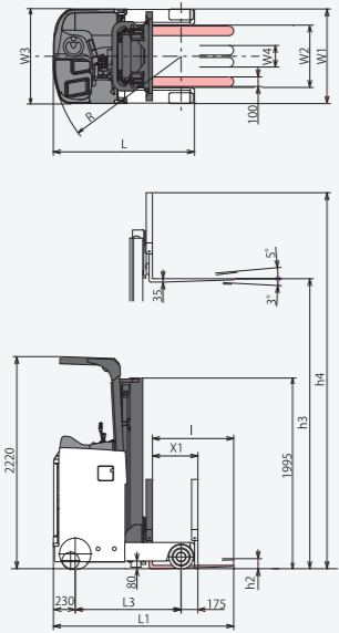
バッテリー前引出し仕様 0.9t~1.2t 積
